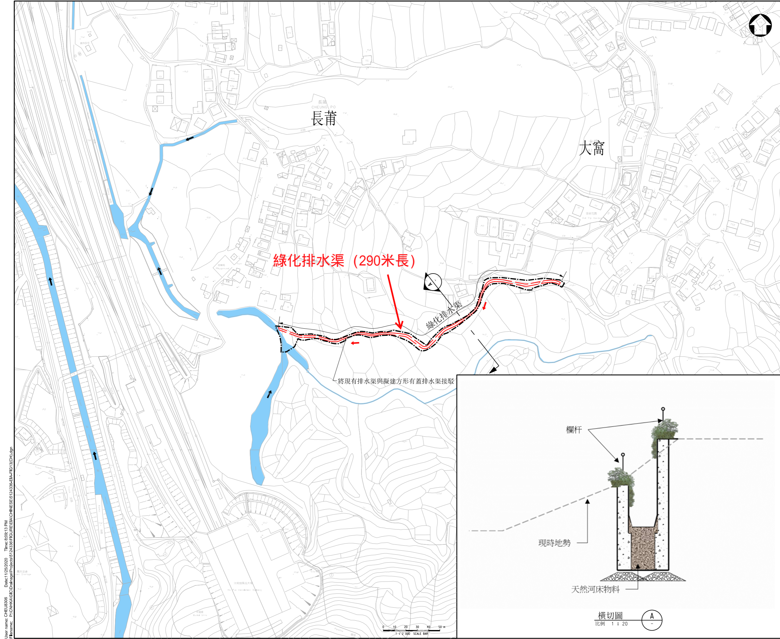
位置圖 N.T.S.
