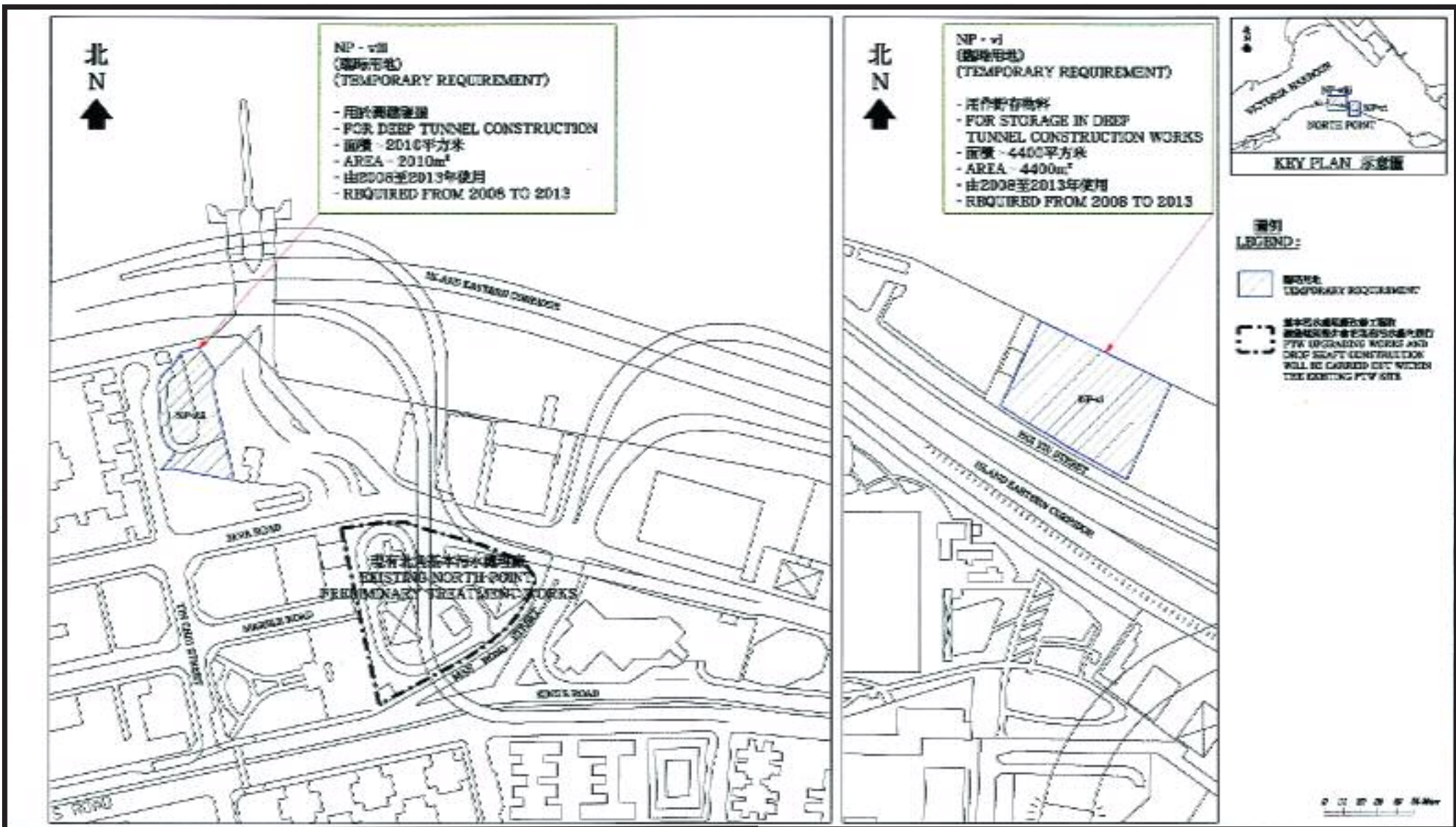
淨化海港計劃第二期甲 在北角的所需工程用地 HARBOUR AREA TREATMENT SCHEME STAGE 2A LAND REQUIREMENT PLAN AT NORTH POINT
