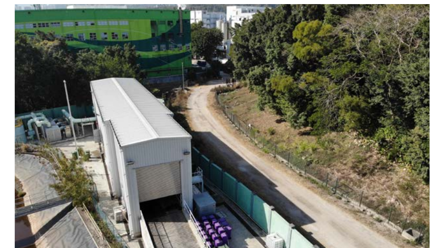
| 用于「厨余、污泥共厌氧消化」试验计划的大埔污水处理厂厨余预处理设施
