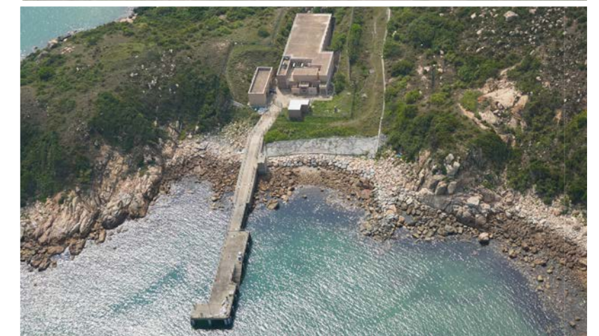
| 小鸦洲低放射性废物贮存设施鸟瞰照片
