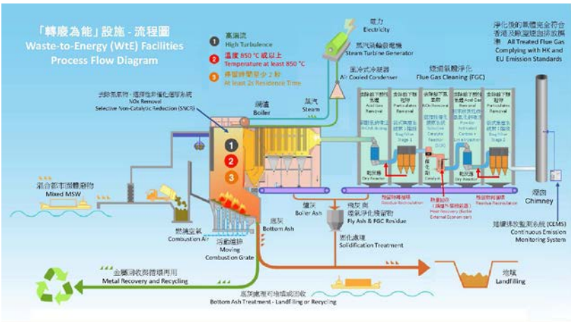
| I·PARK 计划采用的都市固体废物焚化及烟气处理流程
