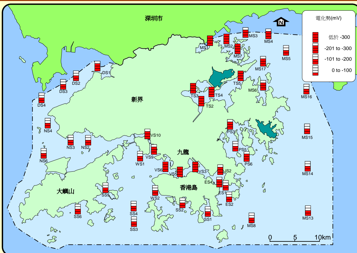
二零零一至二零零五年香港沉積物的電化勢分佈
