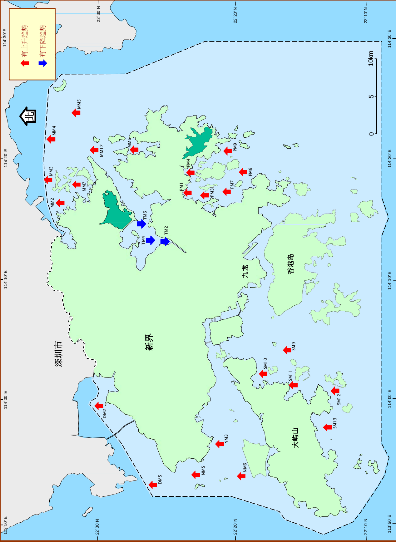
一九八六至二零一三年香港海域叶绿素-a含量的长期变化
