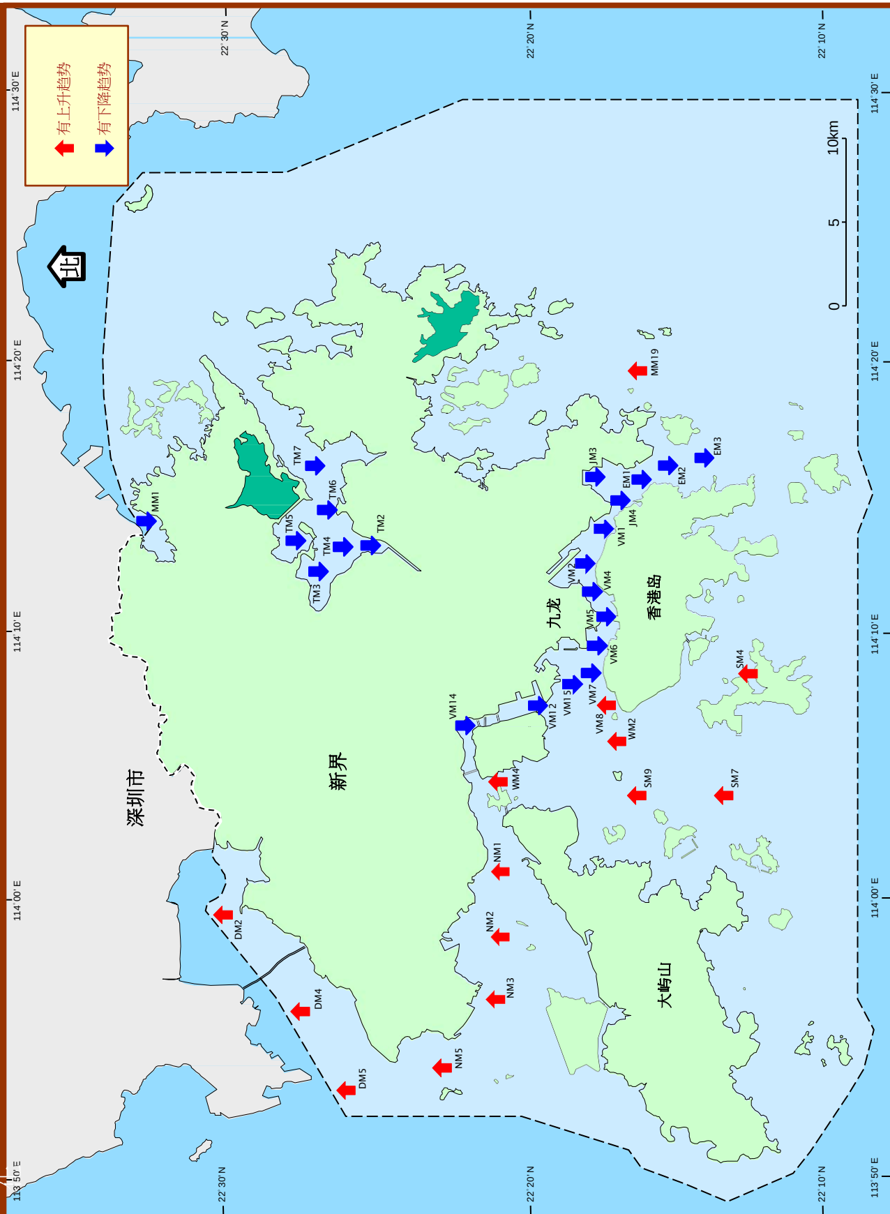
一九八六至二零一三年香港海域氨氮含量的长期变
