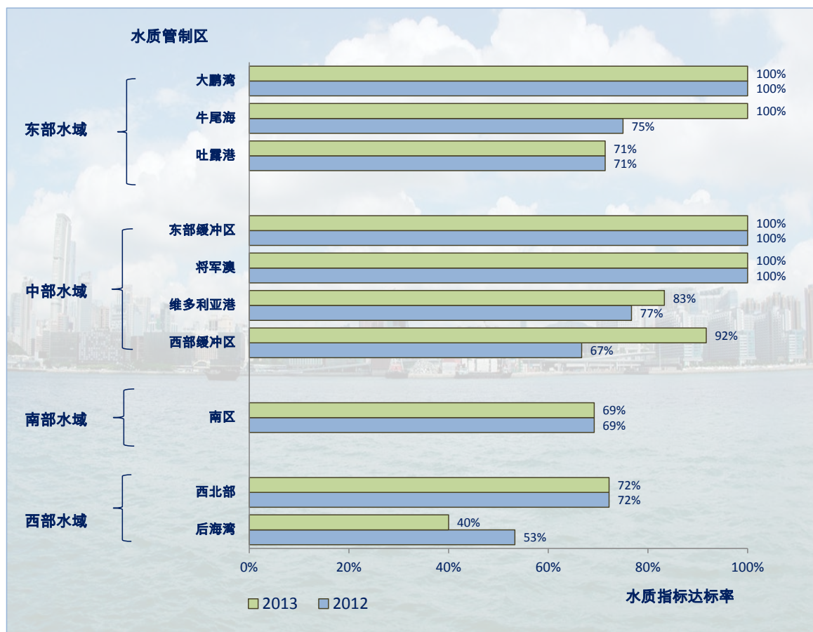
2012 年及 2013 年本港 10 个水质管制区的水质指标达标率
