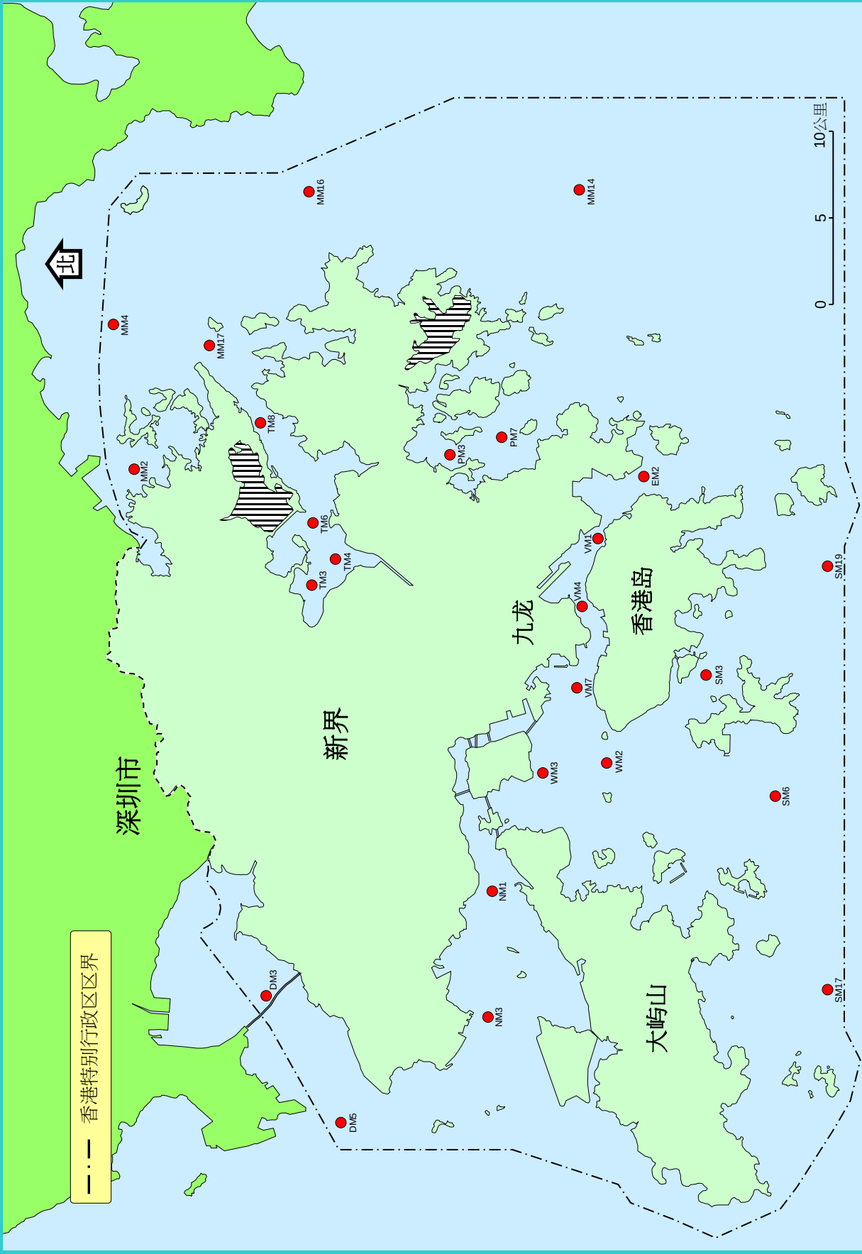
2013年香港海域的浮游植物监测站
