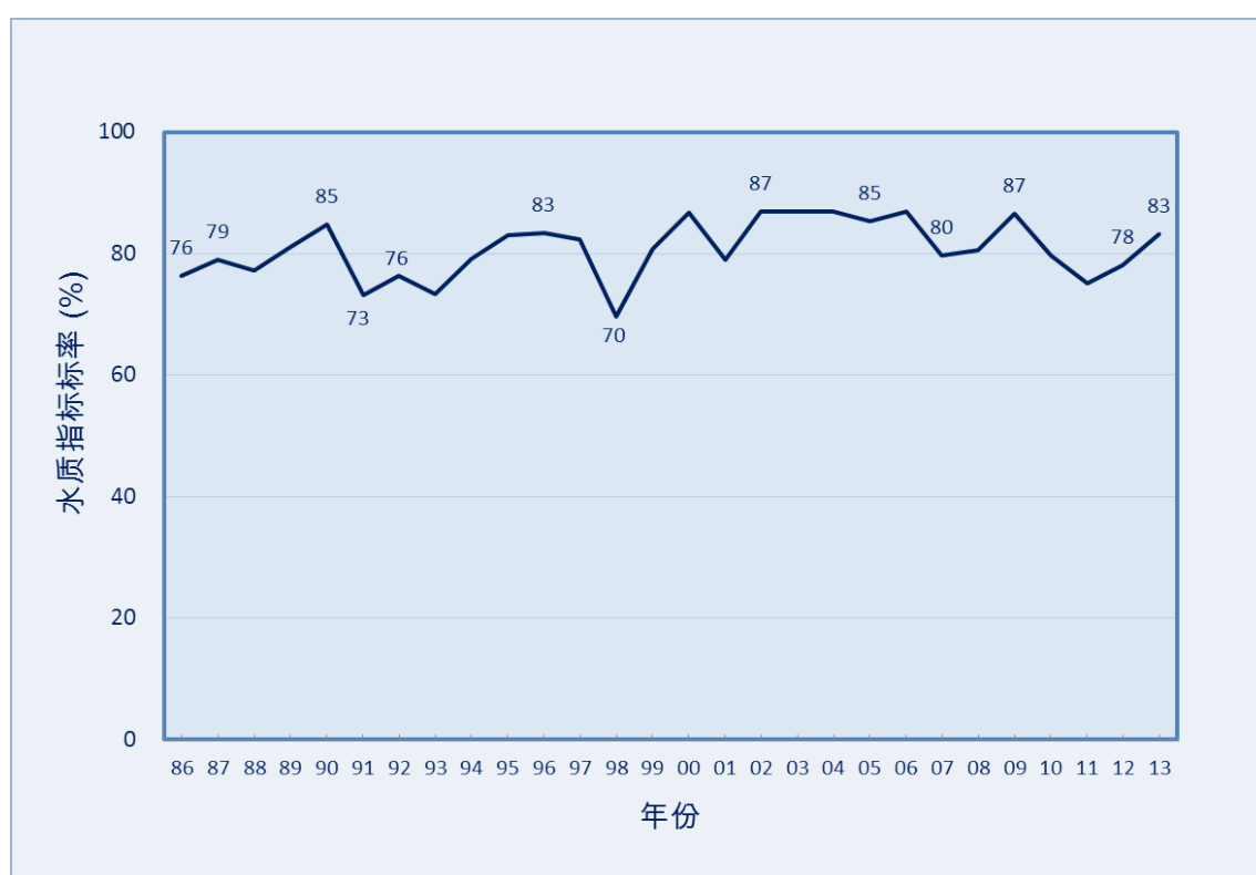
1986年至2013年本港海水水质指标整体达标率
