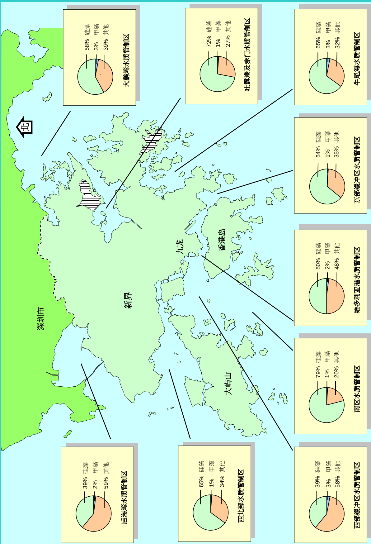
2013年9个水质管制区各浮游植物类别占整体密度百分比
