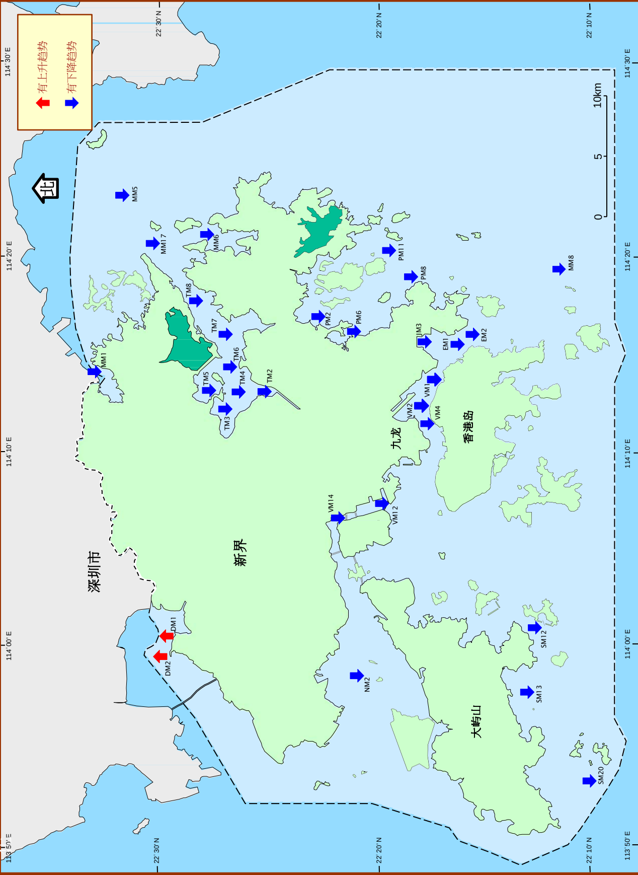
一九八六至二零一三年香港海域五天生化需氧量的长期变
