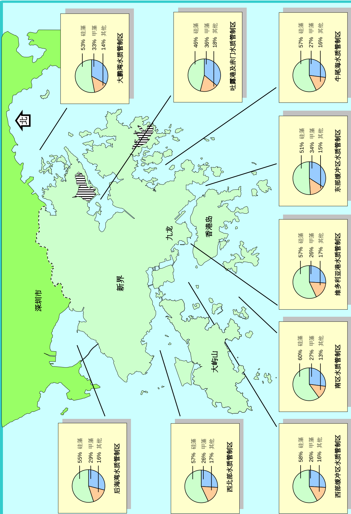
2013年9个水质管制区各浮游植物类别占整体物种数目百分比
