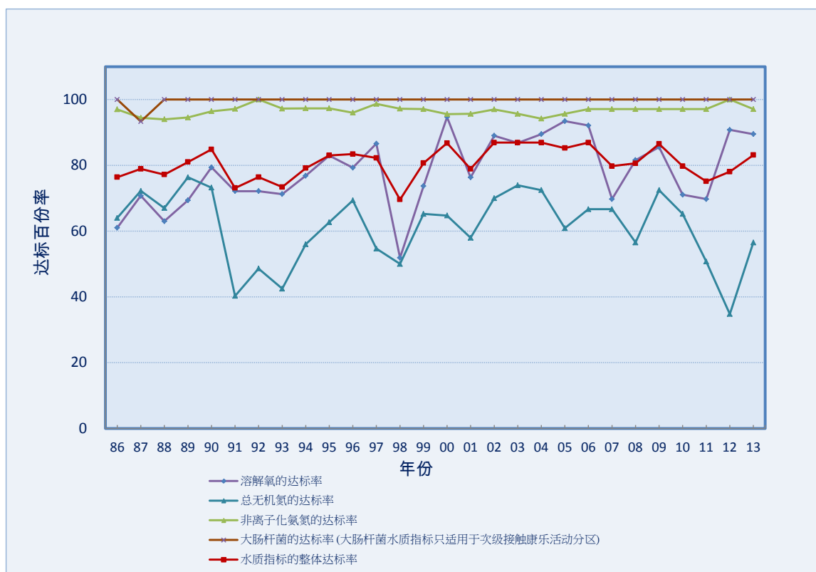
1986 年至 2013 年本港海水水质指标整体达标率及四个重要水质指标达标率
