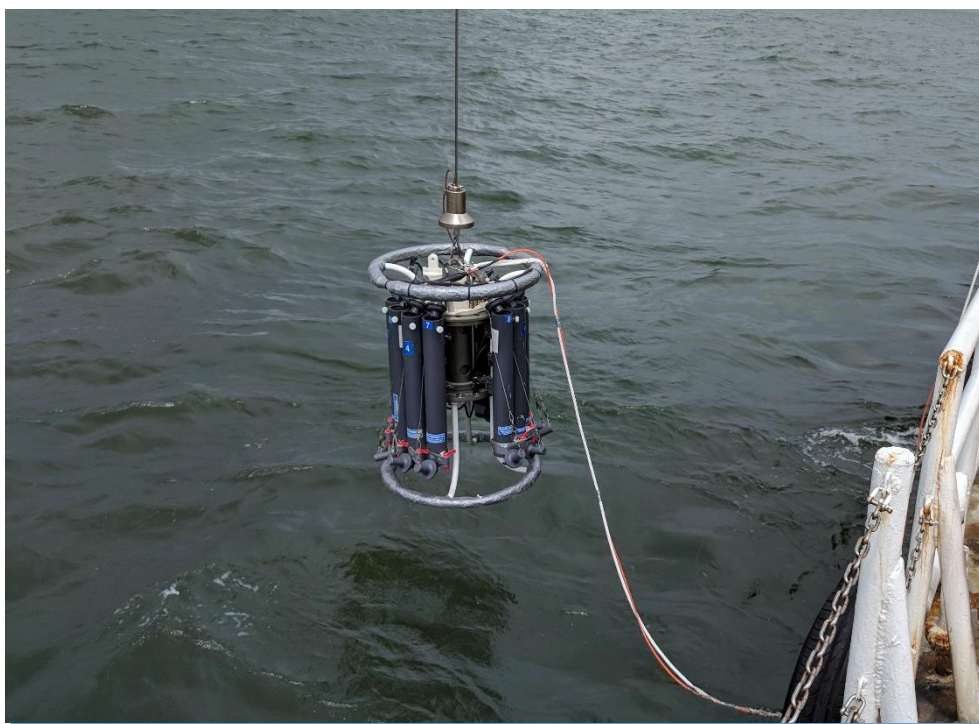
电脑控制的多瓶式采样器
