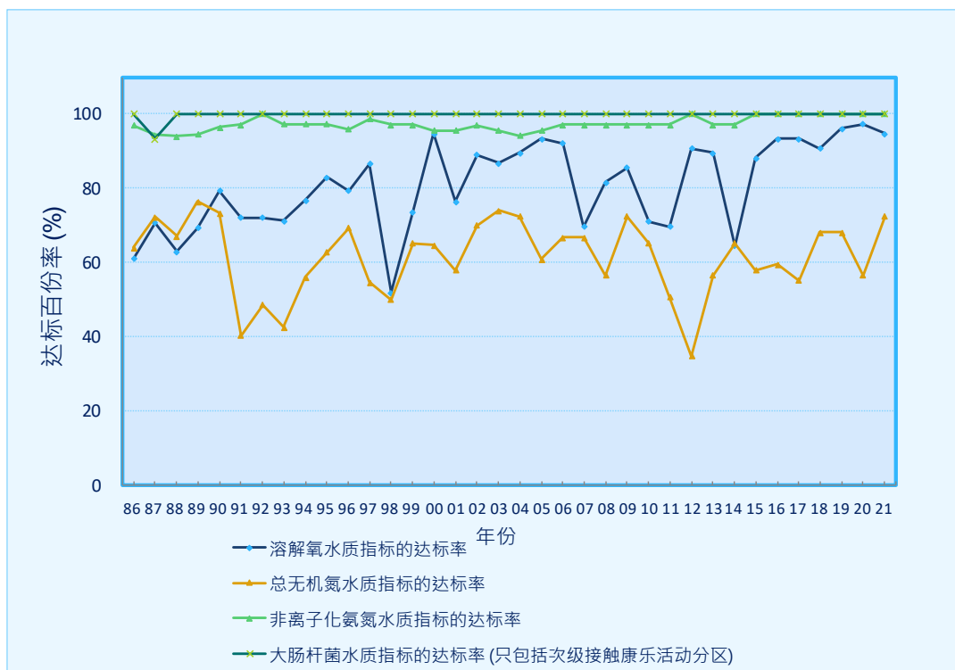
图 2. 4 个主要海水水质指标达标率 (1986-2021 年)
