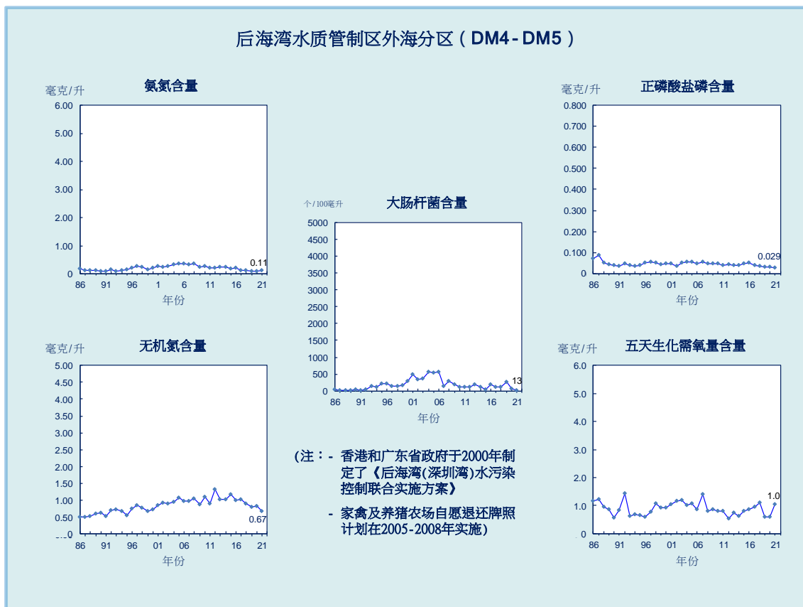
图 22. 后海湾水质管制区外海分区的水质长期趋势 (1986-2021 年)
