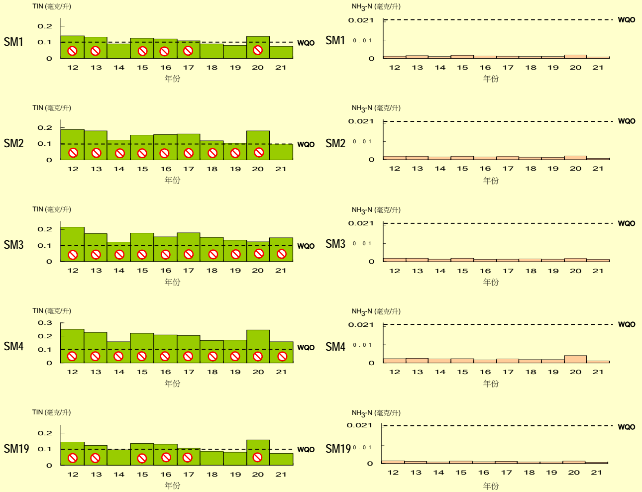
无机氮 (TIN) (水深平均值)
