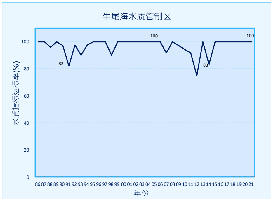
图 7. 牛尾海水水质管制区的水质指标整体达标率 (1986-2021 年)
