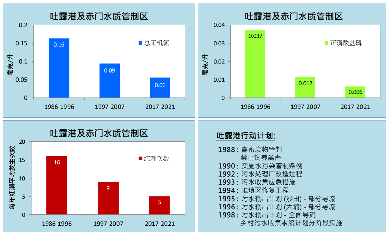
图 28. 吐露港及赤门水质管制区的营养物质含量与红潮次数均明显下降 (1986-2021 年)
