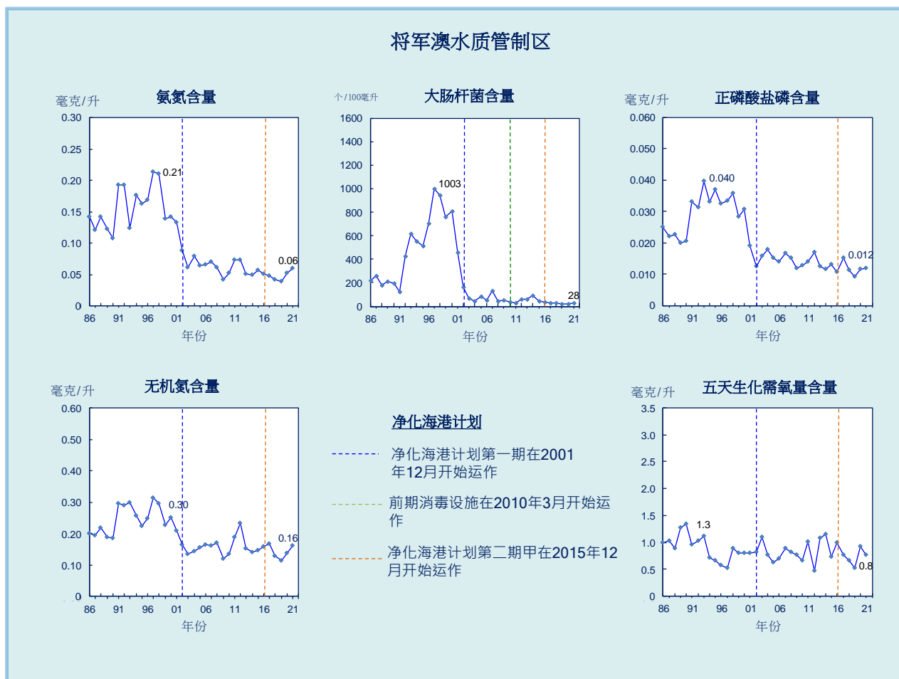
图 17. 将军澳水质管制区的水质长期趋势 (1986-2021 年)
