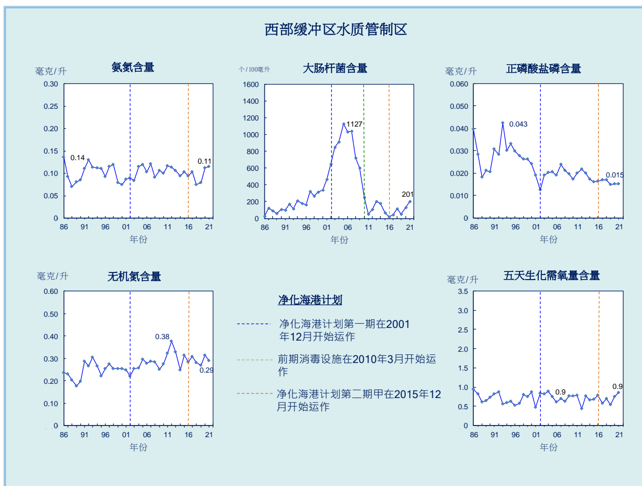
图 19. 西部缓冲区水质管制区的水质长期趋势 (1986-2021 年)
