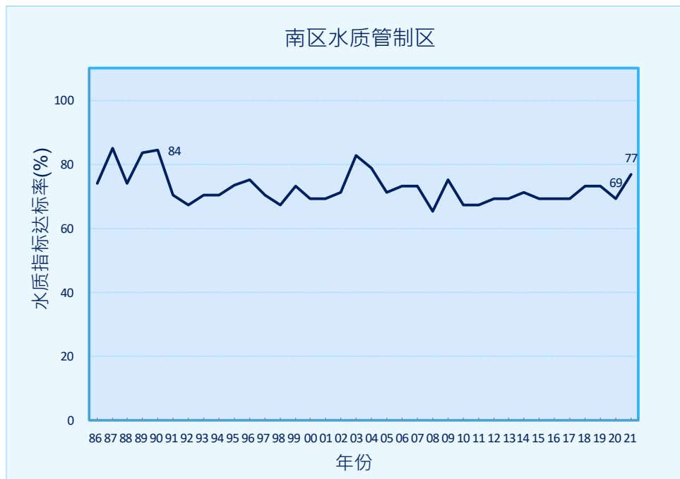
图 25. 南区水质管制区的水质指标整体达标率 (1986-2021 年)
