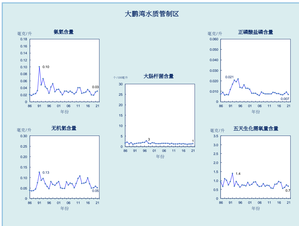
图 6. 大鹏湾水质管制区的水质长期趋势 (1986-2021 年)
