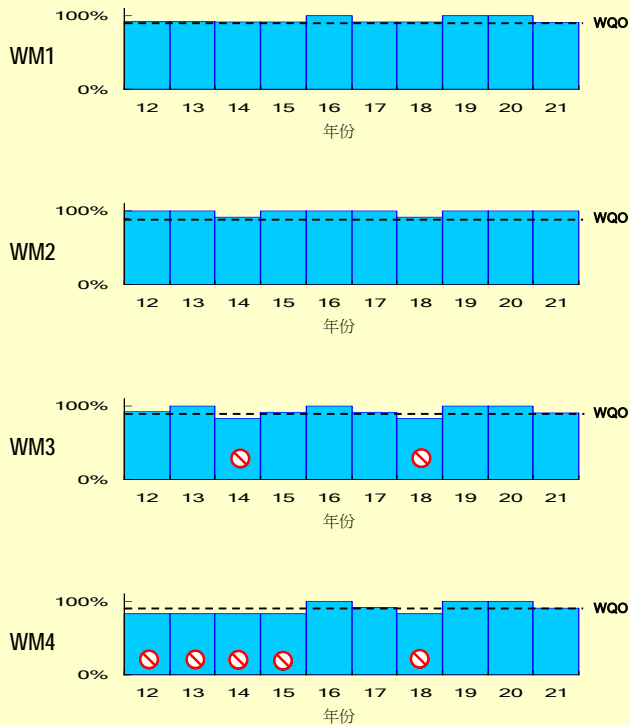
溶解氧 (DO) (水深平均值)
