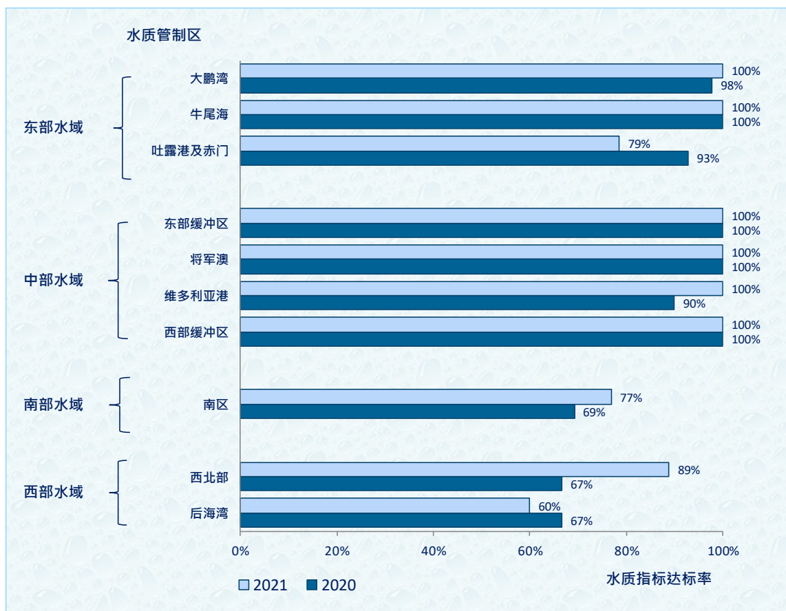
图 3. 10 个水质管制区的水质指标达标率 (2020 年及 2021 年)
