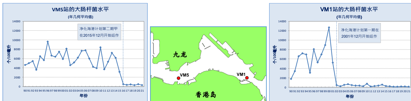
图11. 维多利亚港水质管制区中部 (VM5) 及东部 (VM1) 的大肠杆菌水平 (1990-2021年)
