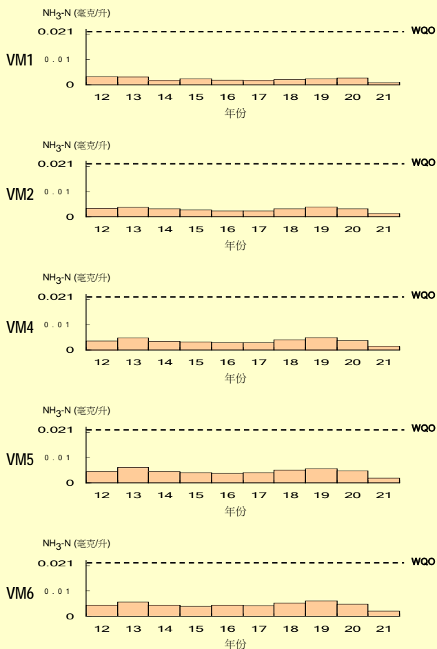
非离子氨气 (NH 3 -N) (水深平均值)
