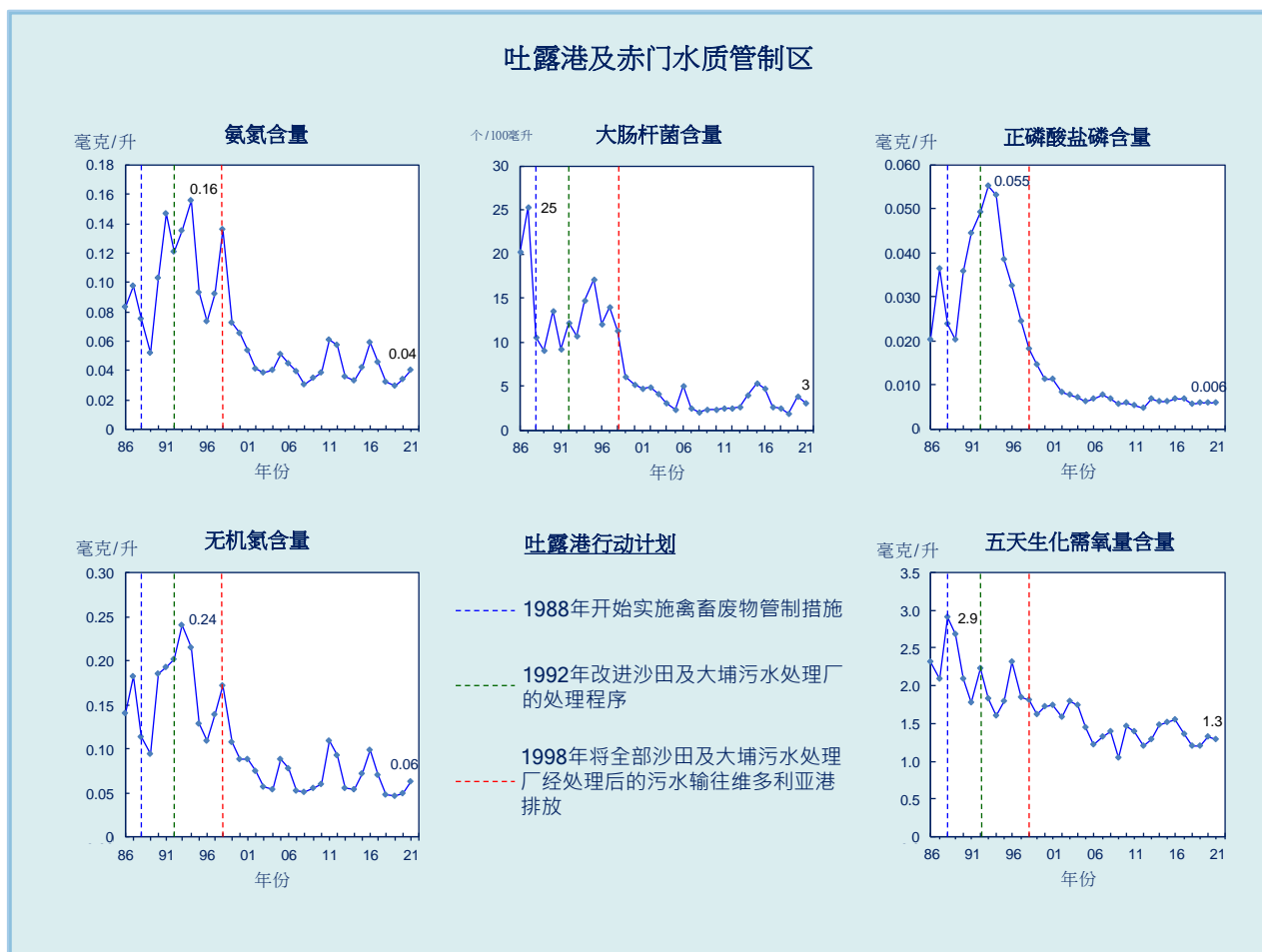
图 10. 吐露港及赤门水质管制区的水质长期趋势 (1986-2021 年)
