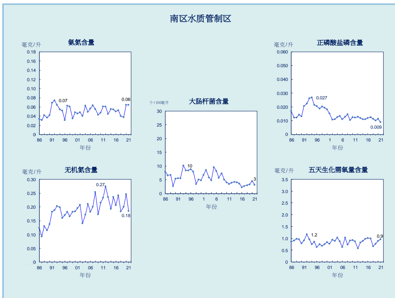
图 26. 南区水质管制区的水质长期趋势 (1986-2021 年)
