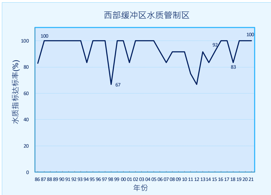
图 18. 西部缓冲区水质管制区的水质指标整体达标率 (1986-2021 年)
