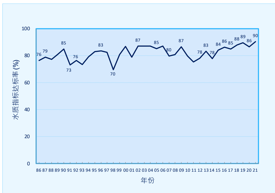
图 1. 香港海水水质指标整体达标率（1986-2021 年）
