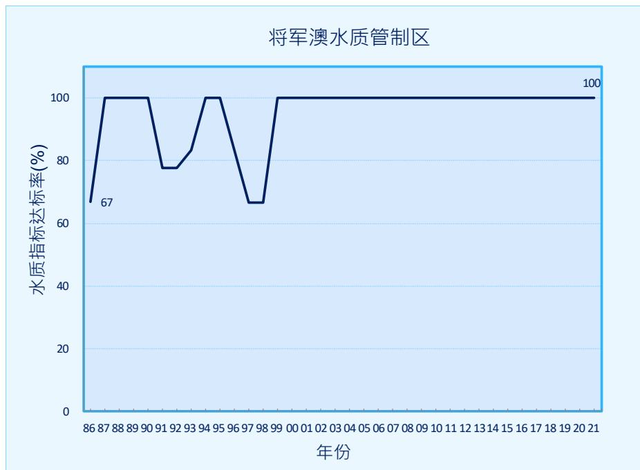
图 16. 将军澳水质管制区的水质指标整体达标率 (1986-2021 年)
