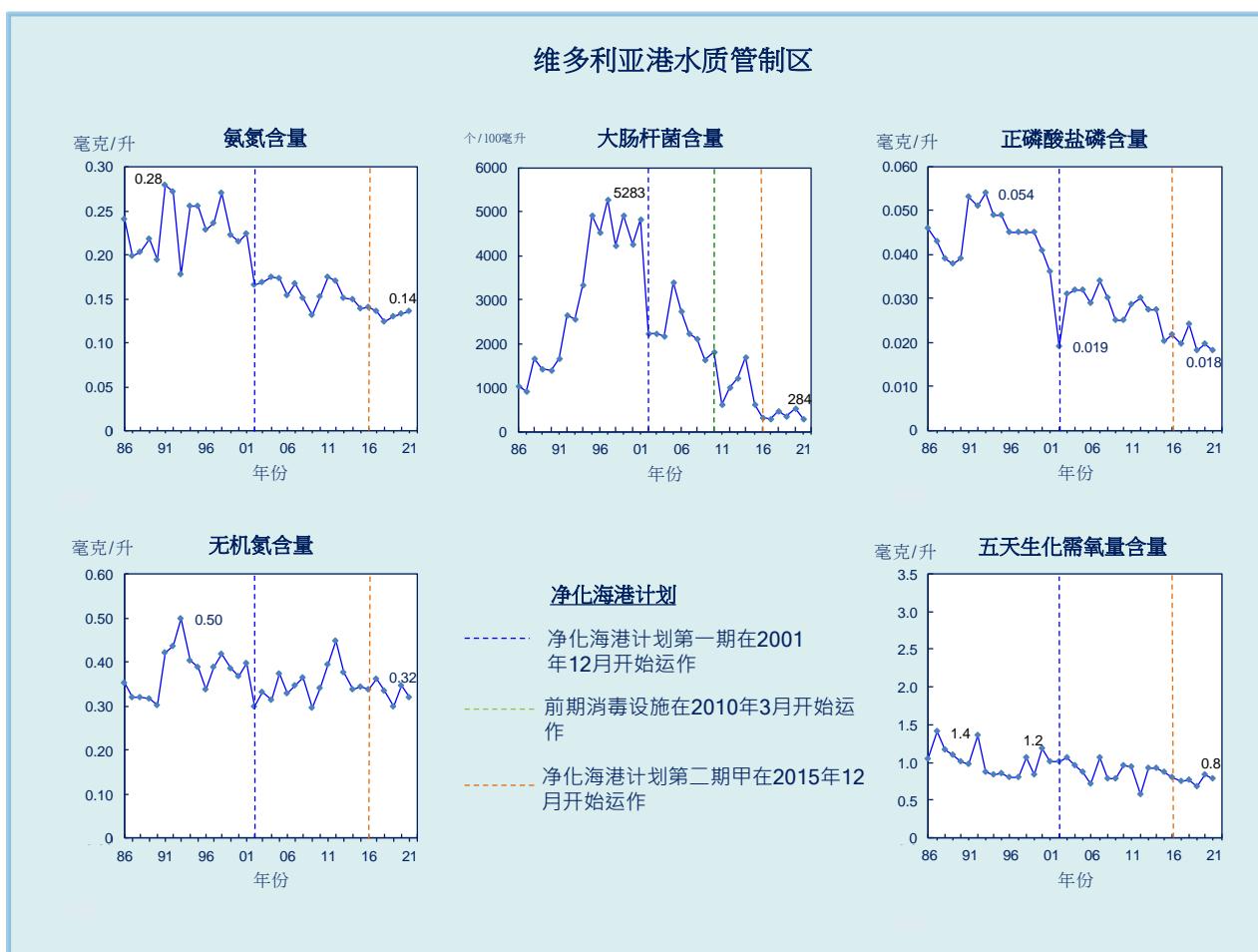
图 13. 维多利亚港水质管制区的水质长期趋势 (1986-2021年)
