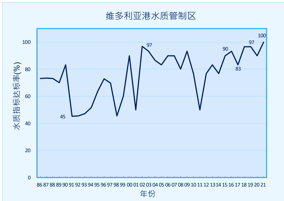
图 12. 维多利亚港水质管制区的水质指标整体达标率 (1986-2021 年)
