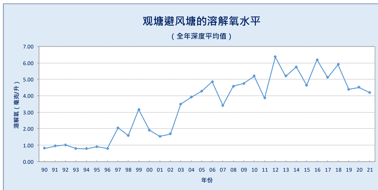
图 27. 观塘避风塘的水中溶解氧含量呈长期改善趋势（1990-2021 年）
