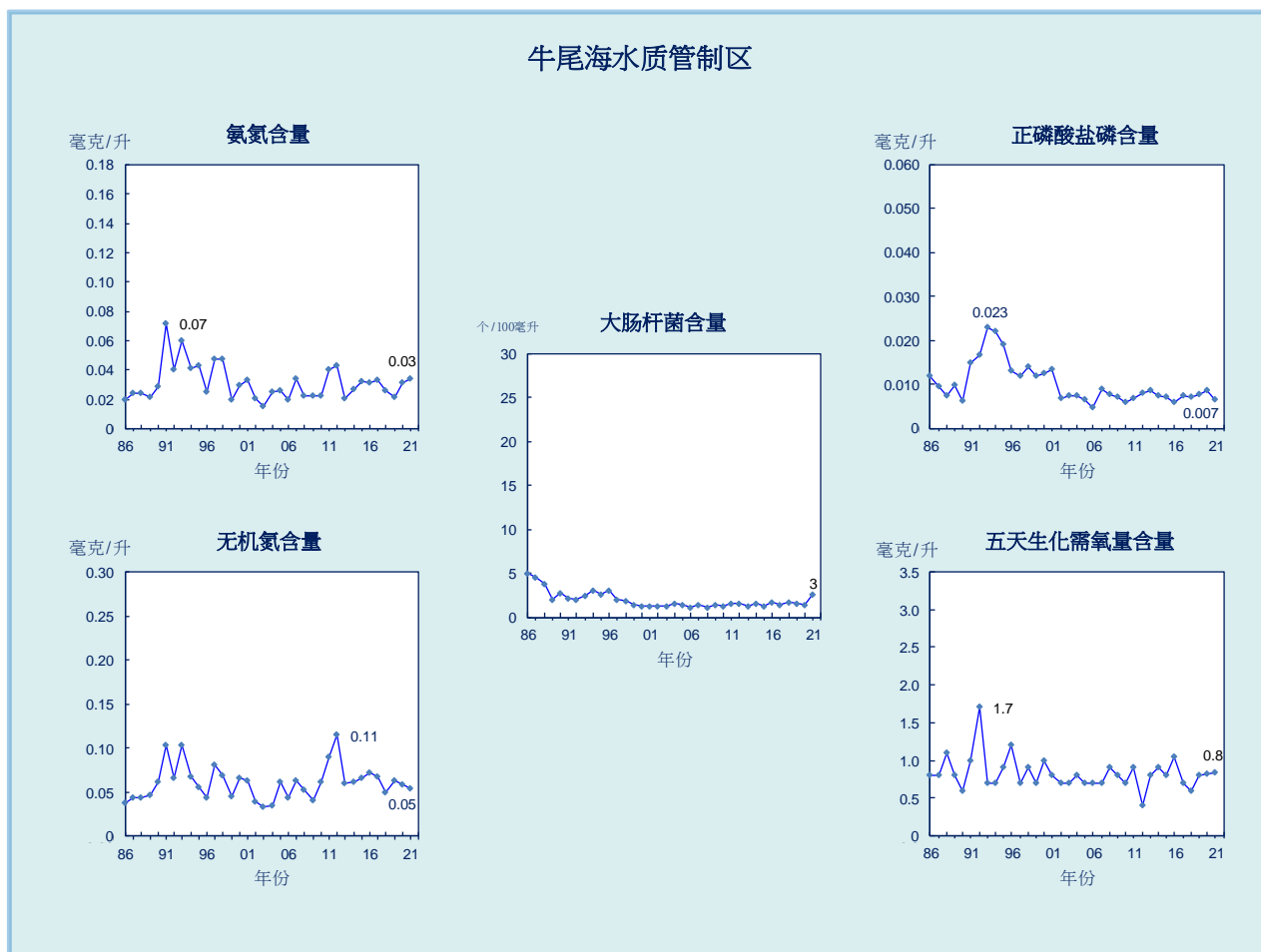
图 8. 牛尾海水水质管制区的水质长期趋势 (1986-2021年)
