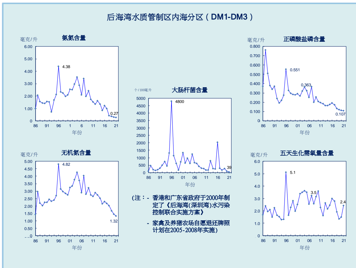
图 21. 后海湾水质管制区内海分区的水质长期趋势 (1986-2021 年)
