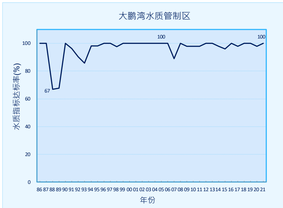
图 5. 大鹏湾水质管制区的水质指标整体达标率 (1986-2021 年)
