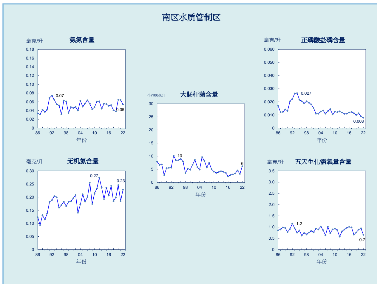
图 26. 南区水质管制区的水质长期趋势 (1986-2022 年)
