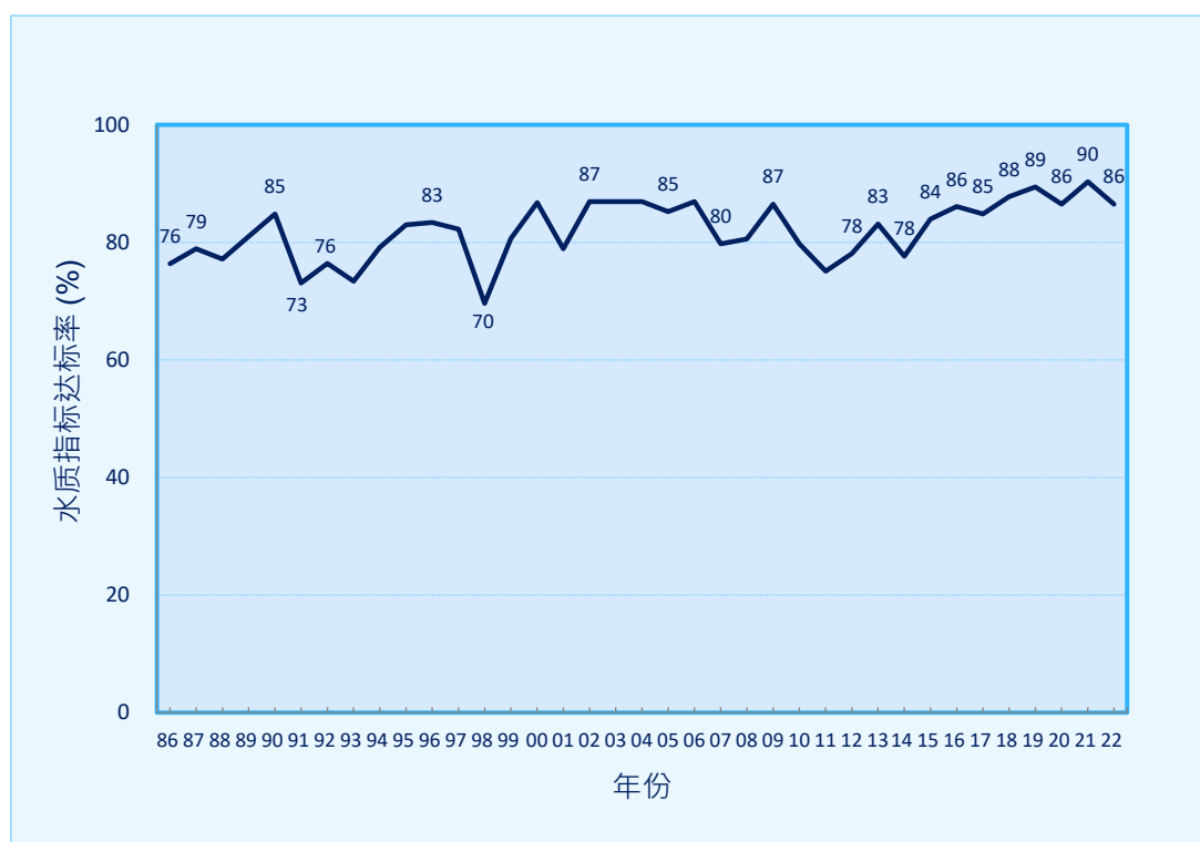
图 1. 香港海水水质指标整体达标率（1986-2022 年）
