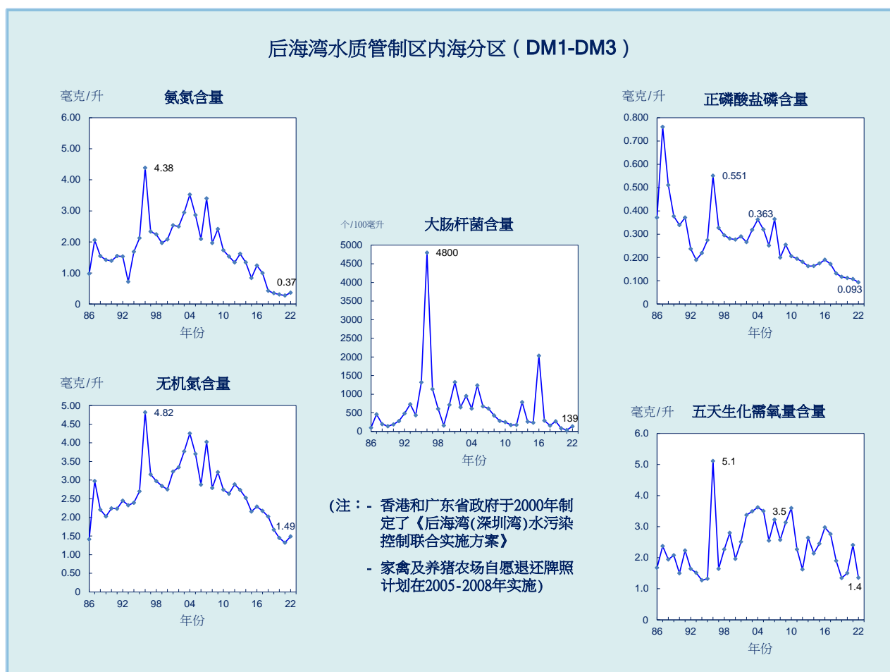
图 21. 后海湾水质管制区内海分区的水质长期趋势 (1986-2022 年)
