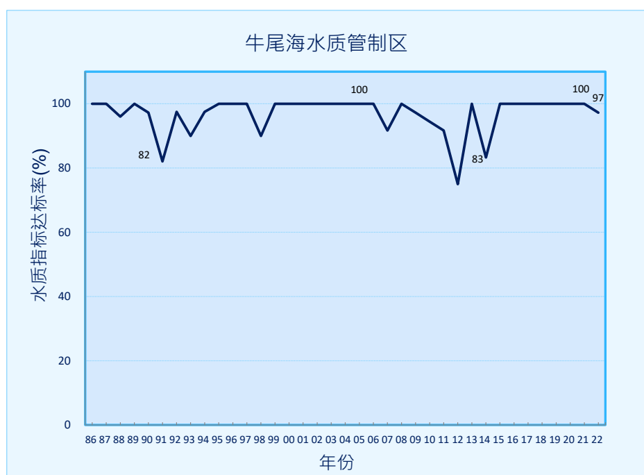
图7. 牛尾海水质管制区的水质指标整体达标率（1986-2022年）
