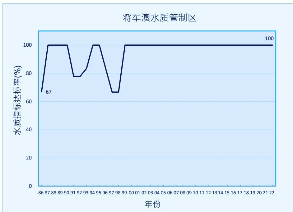
图 16. 将军澳水质管制区的水质指标整体达标率 (1986-2022 年)
