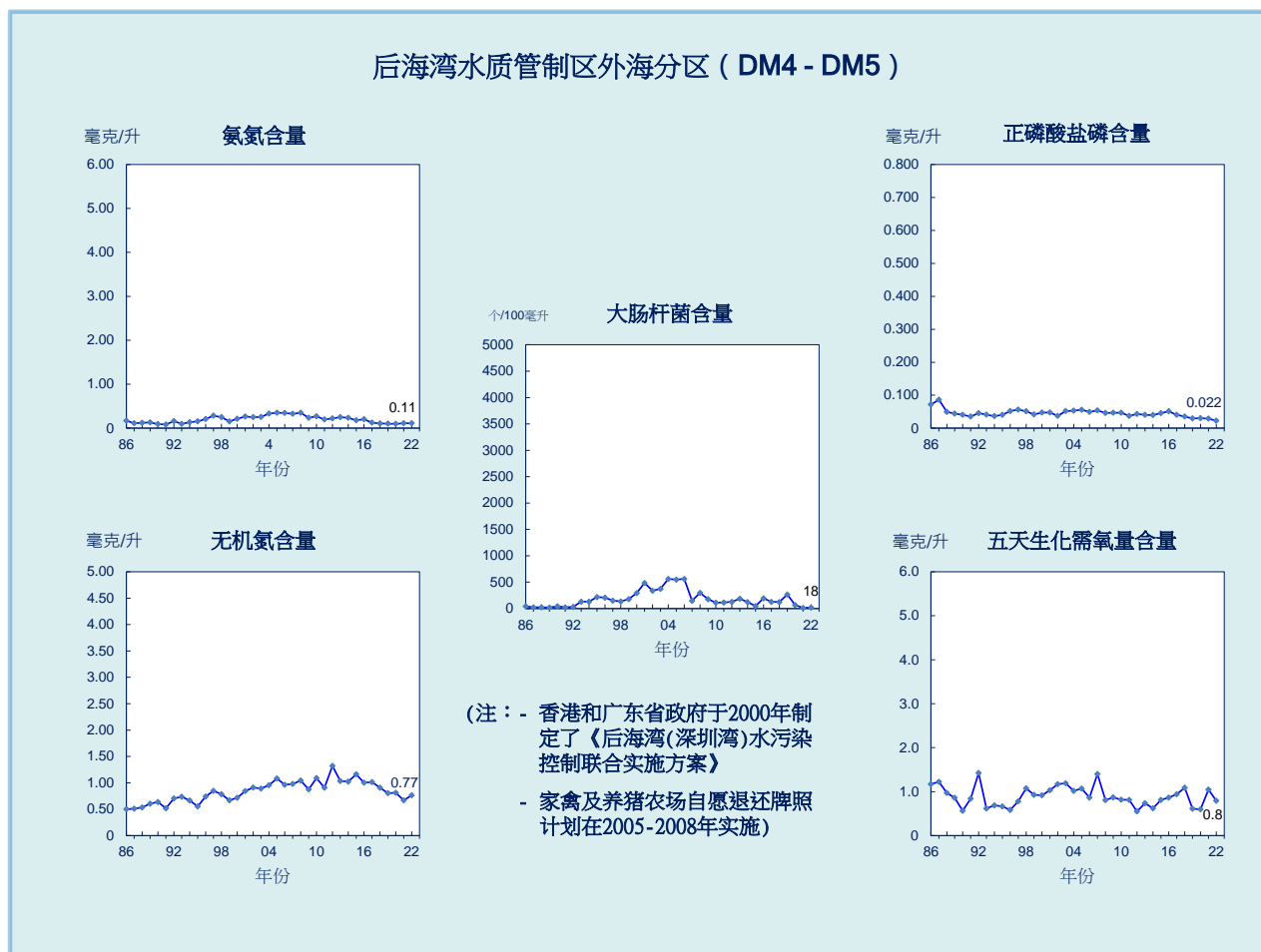
图 22. 后海湾水质管制区外海分区的水质长期趋势 (1986-2022 年)
