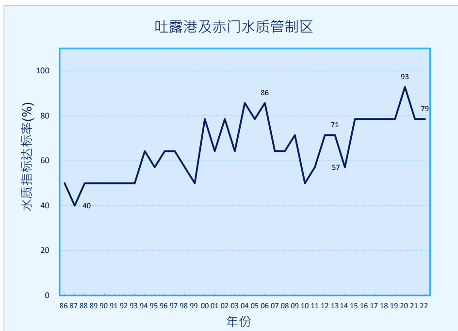
图 9. 吐露港及赤门水质管制区的水质指标整体达标率 (1986-2022 年)
