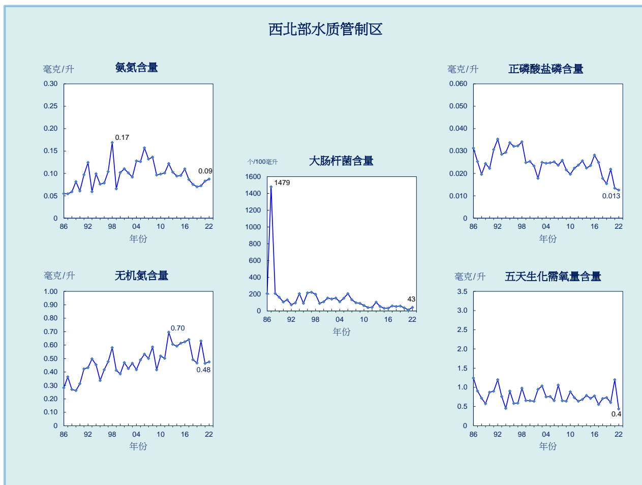
图 24. 西北部水质管制区的水质长期趋势 (1986-2022 年)
