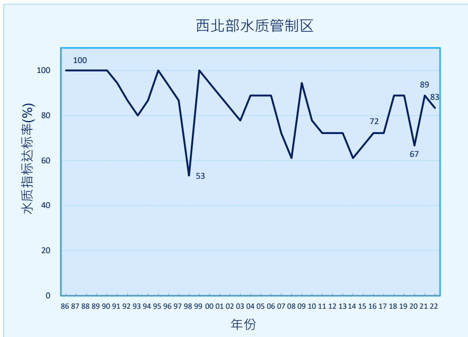
图 23. 西北部水质管制区的水质指标整体达标率 (1986-2022 年)
