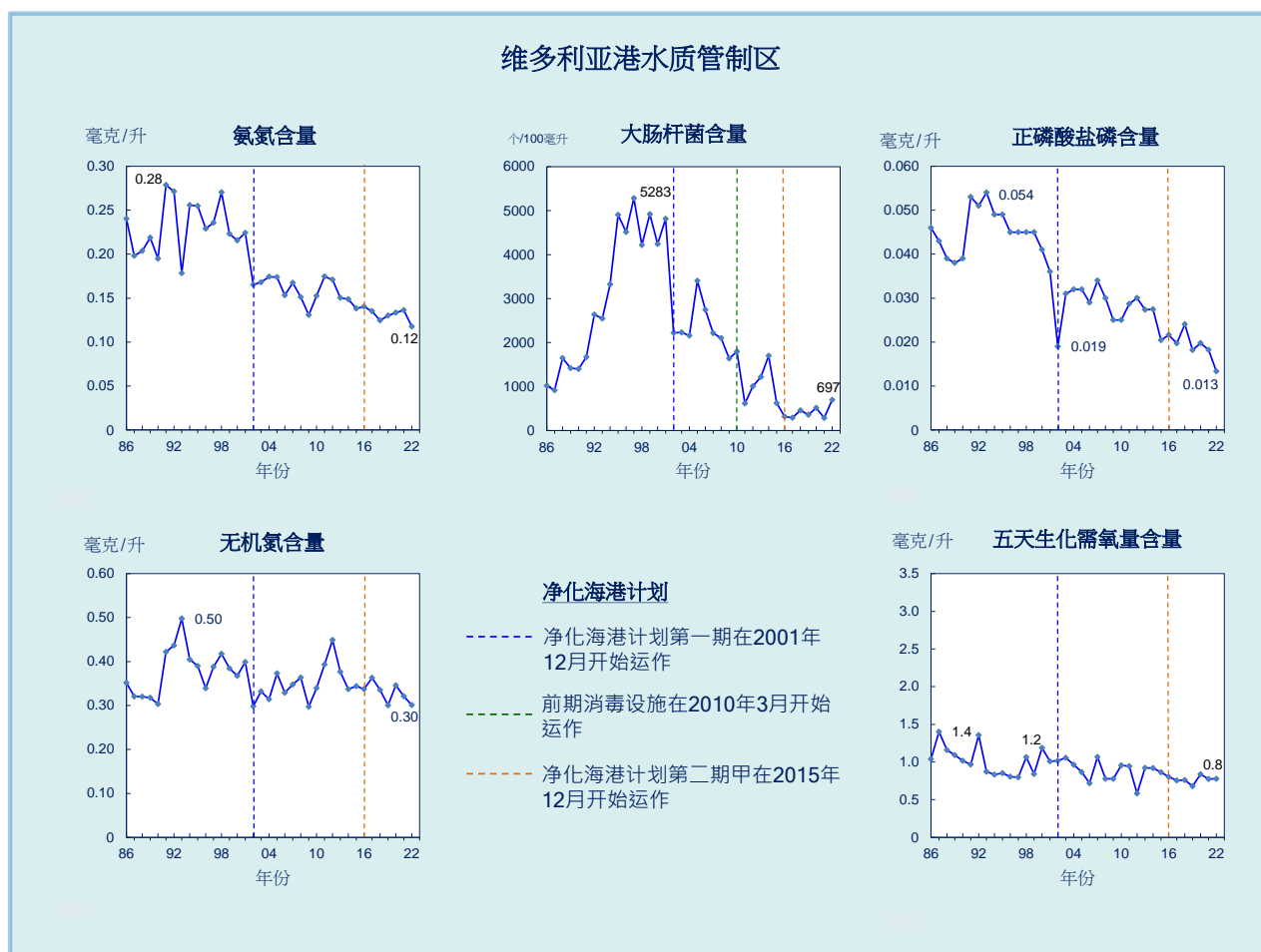
图13. 维多利亚港水质管制区的水质长期趋势（1986-2022年）
