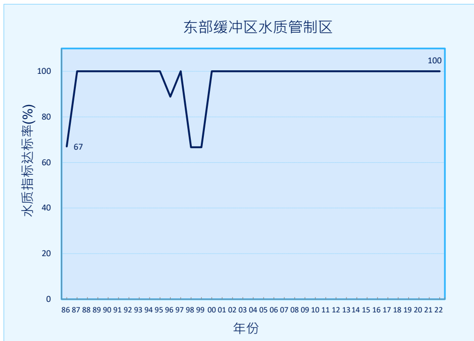
图 14. 东部缓冲区水质管制区的水质指标整体达标率 (1986-2022 年)
