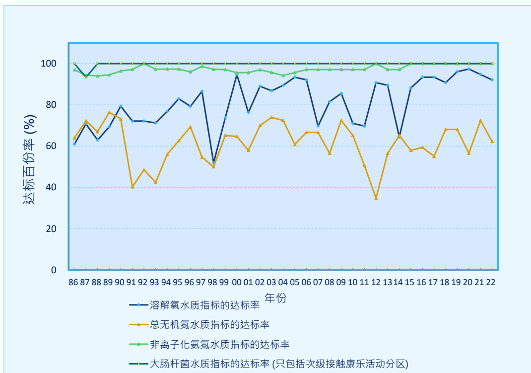
图 2. 4 个主要海水水质指标达标率 (1986-2022 年)
