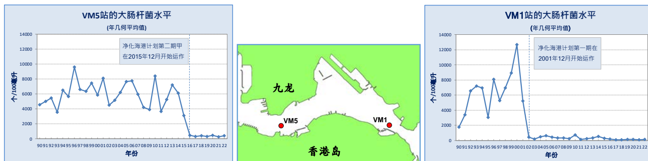
图 11. 维多利亚港水质管制区中部 (VM5) 及东部 (VM1) 的大肠杆菌水平 (1990-2022 年)
