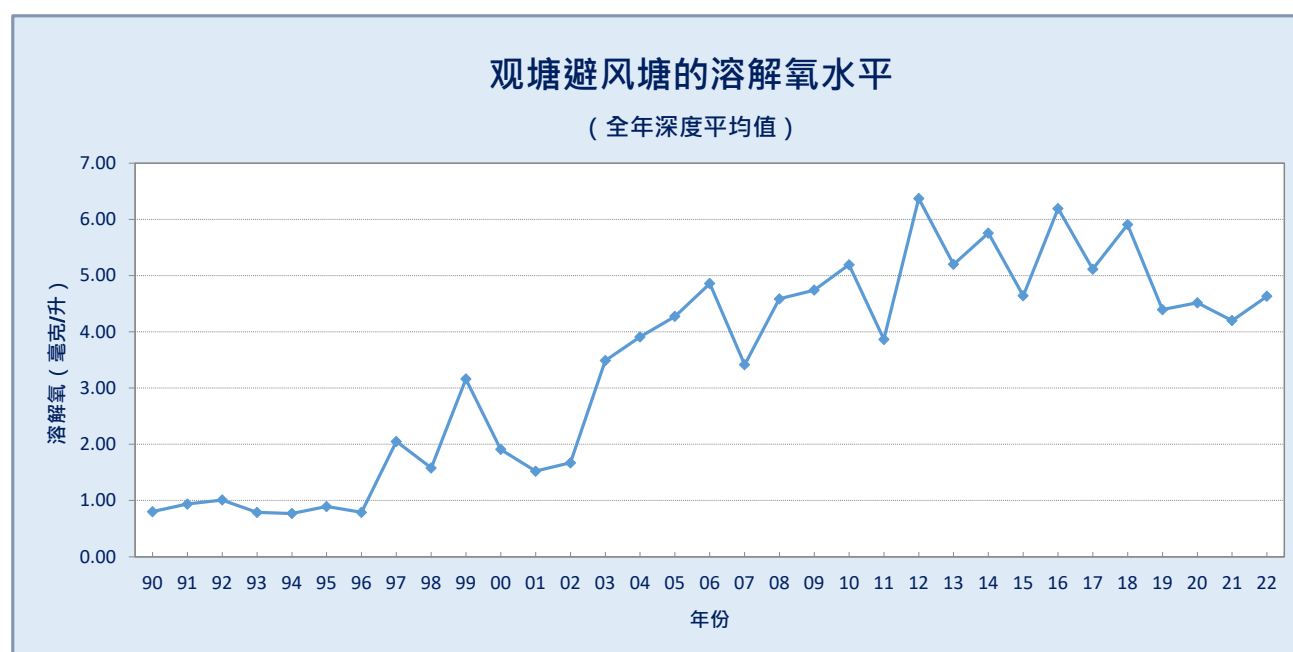
图 27. 观塘避风塘的水中溶解氧含量呈长期改善趋势（1990-2022 年）
