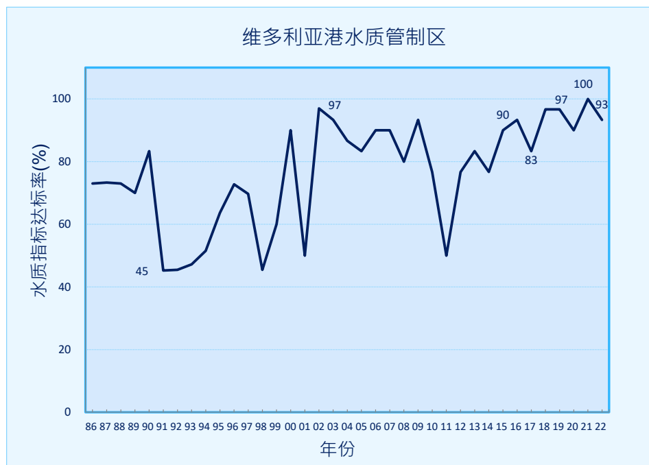
图 12. 维多利亚港水质管制区的水质指标整体达标率 (1986-2022 年)
