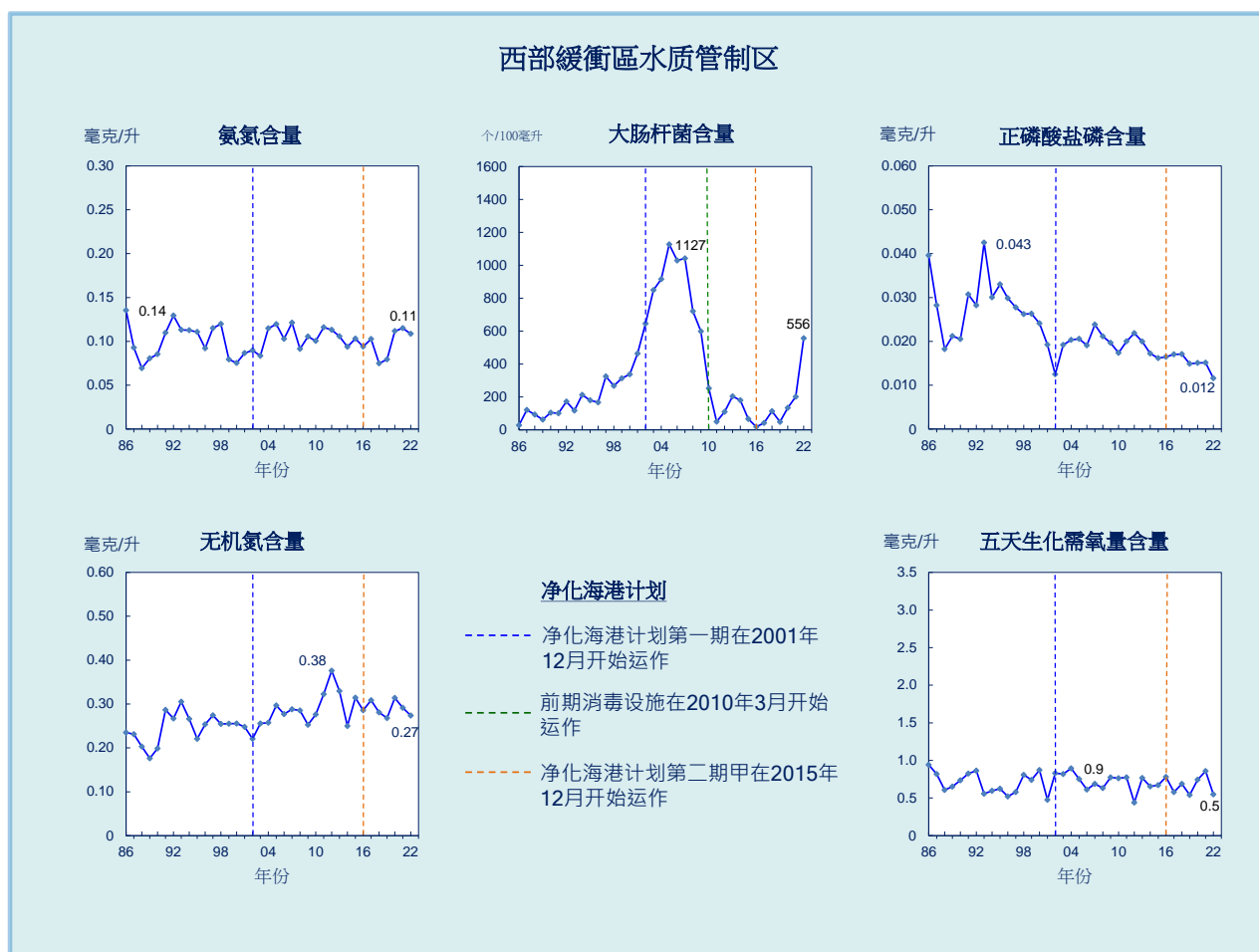
图 19. 西部缓冲区水质管制区的水质长期趋势 (1986-2022 年)
