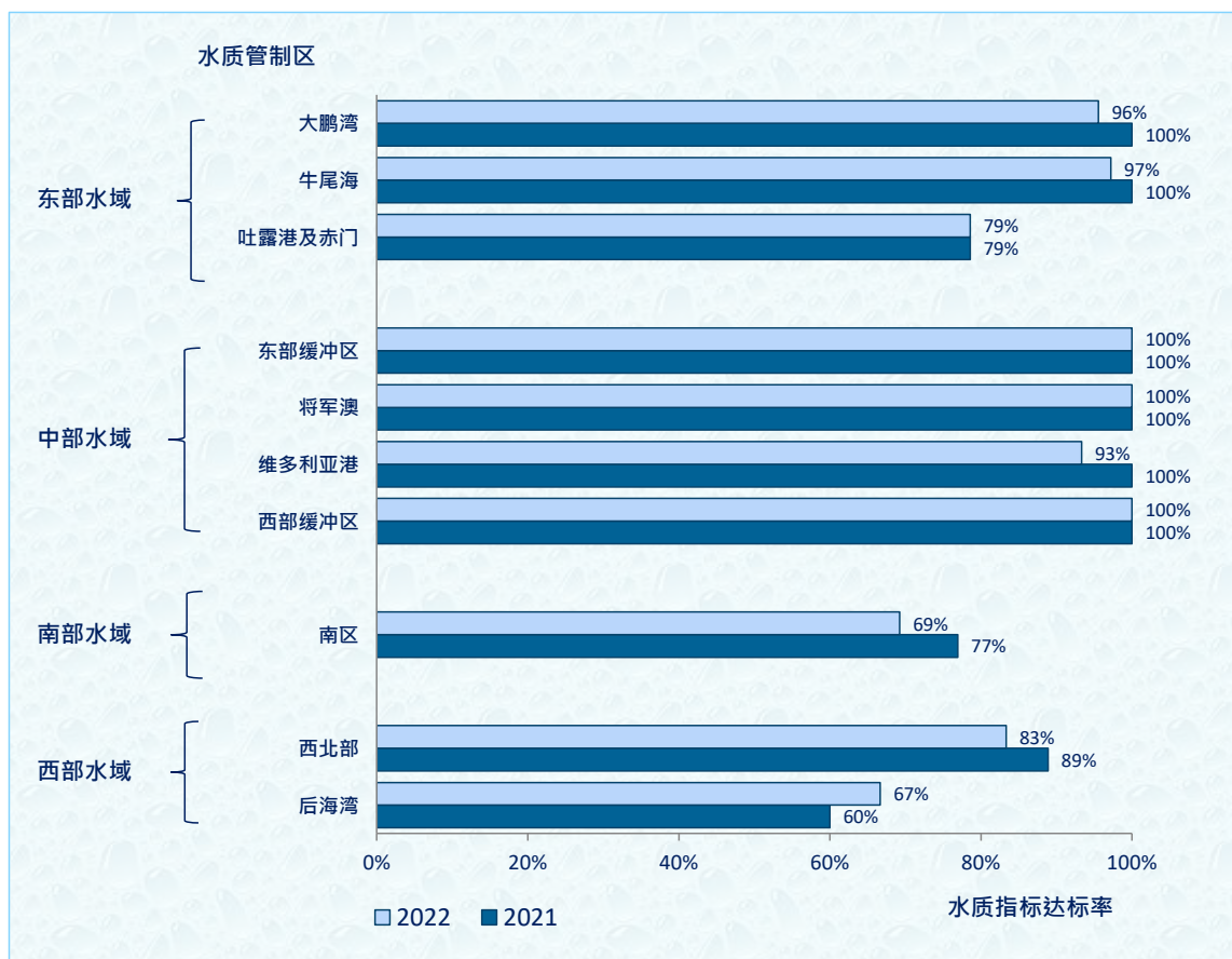
图 3. 10 个水质管制区的水质指标达标率 (2020 年及 2022 年)
