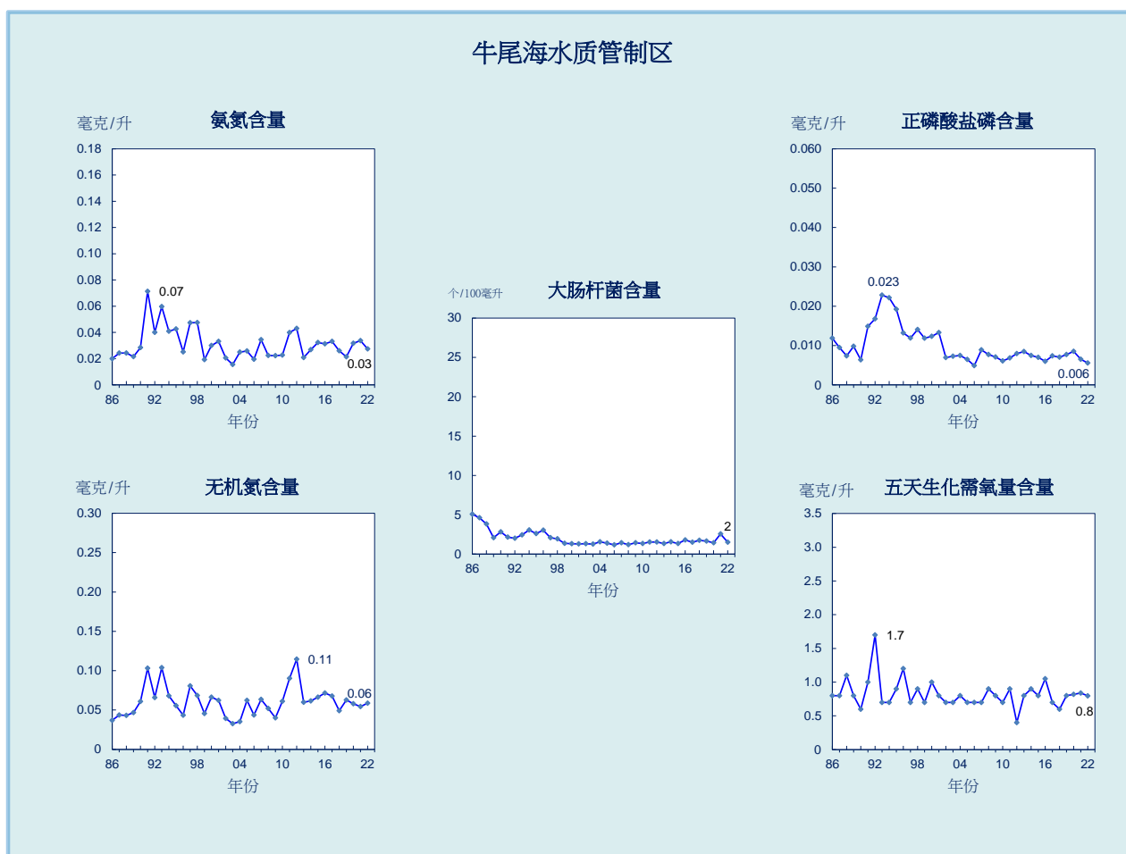
图8. 牛尾海水质管制区的水质长期趋势 (1986-2022年)
