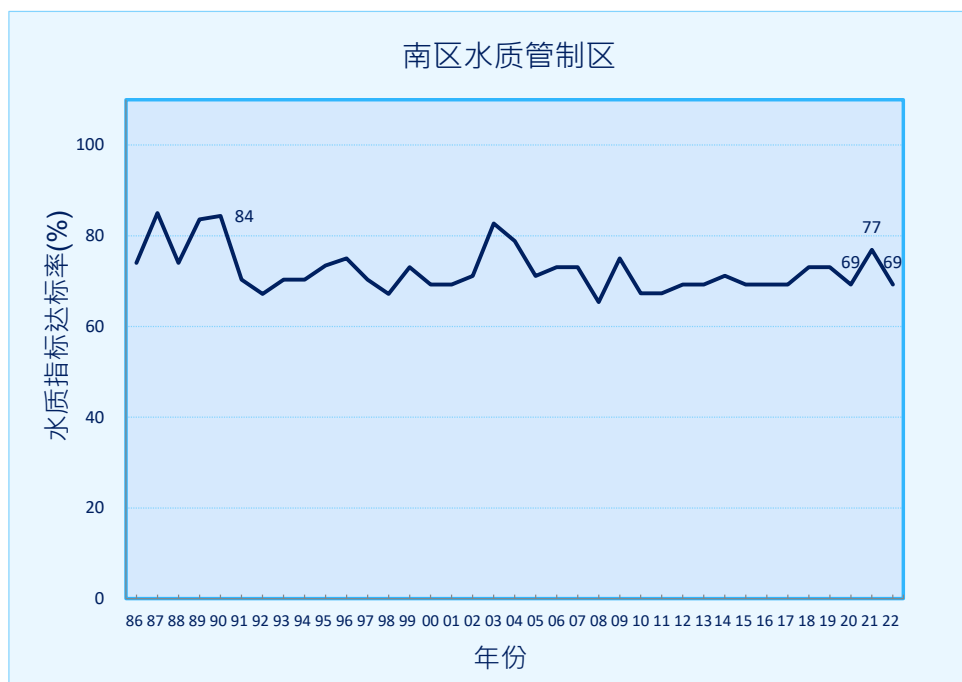
图 25. 南区水质管制区的水质指标整体达标率 (1986-2022 年)
