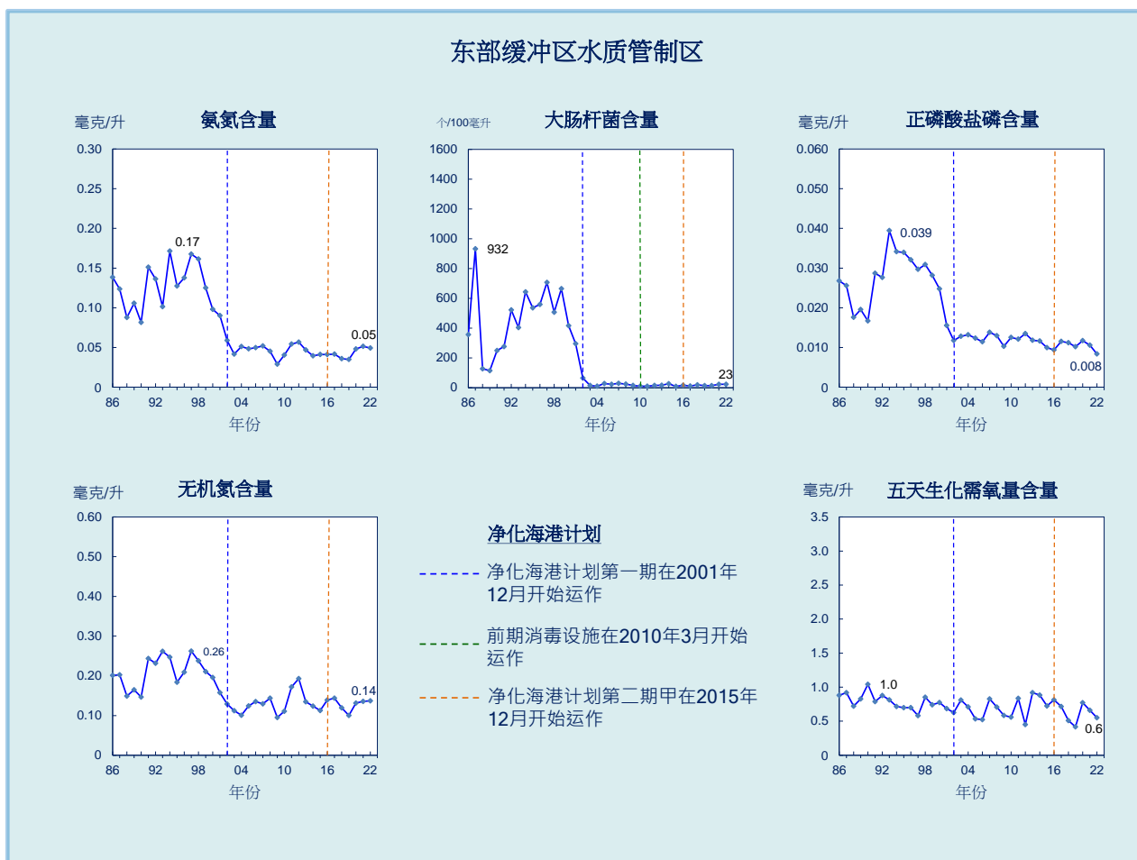
图 15. 东部缓冲区水质管制区的水质长期趋势 (1986-2022 年)
