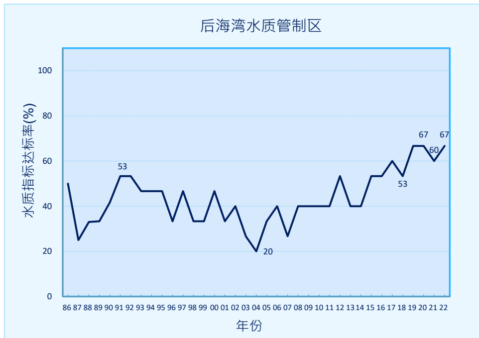
图 20. 后海湾水质管制区的水质指标整体达标率 (1986-2022 年)
