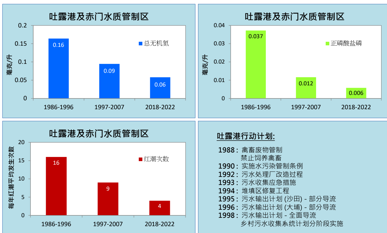
图 28. 吐露港及赤门水质管制区的营养物含量与红潮次数均明显下降 (1986-2022 年)
