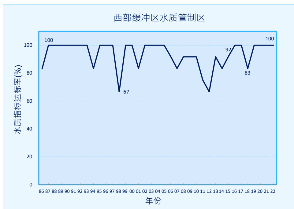
图 18. 西部缓冲区水质管制区的水质指标整体达标率（1986-2022 年）
