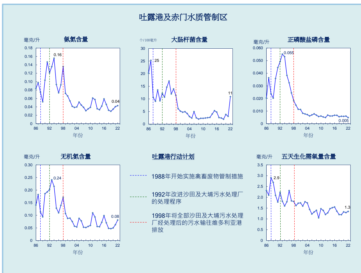
图 10. 吐露港及赤门水质管制区的水质长期趋势 (1986-2022 年)
