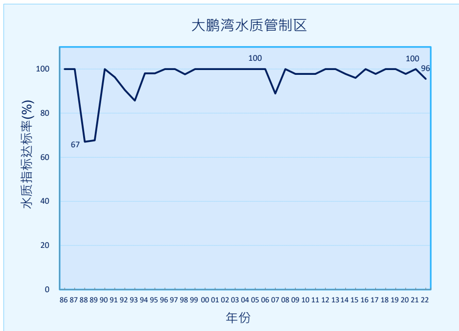
图 5. 大鹏湾水质管制区的水质指标整体达标率 (1986-2022 年)
