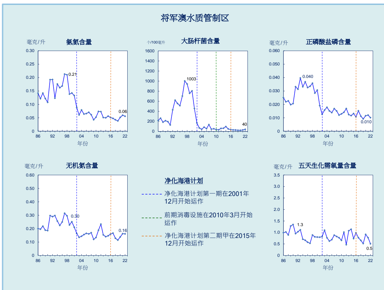
图 17. 将军澳水质管制区的水质长期趋势 (1986-2022 年)
