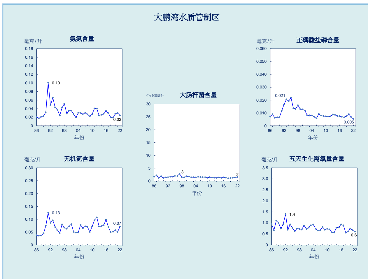
图 6. 大鹏湾水质管制区的水质长期趋势 (1986-2022 年)
