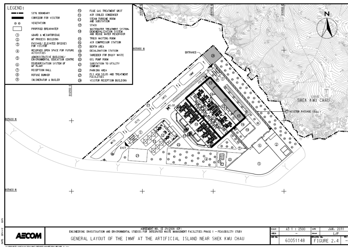
圖 5 -擬建的綜合廢物管理設施第一期佈置圖(毗鄰石鼓洲的人工島)
