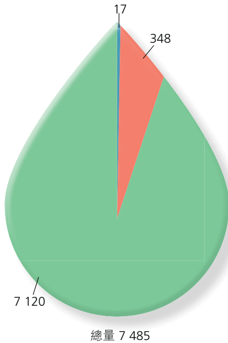
昂坪污水處理廠的碳足跡 (以每公噸二氧化碳當量計)
