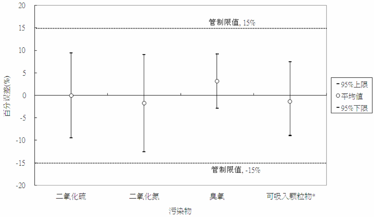
图 2：2008 年粤港珠江三角洲区域空气监控网络的准确度
