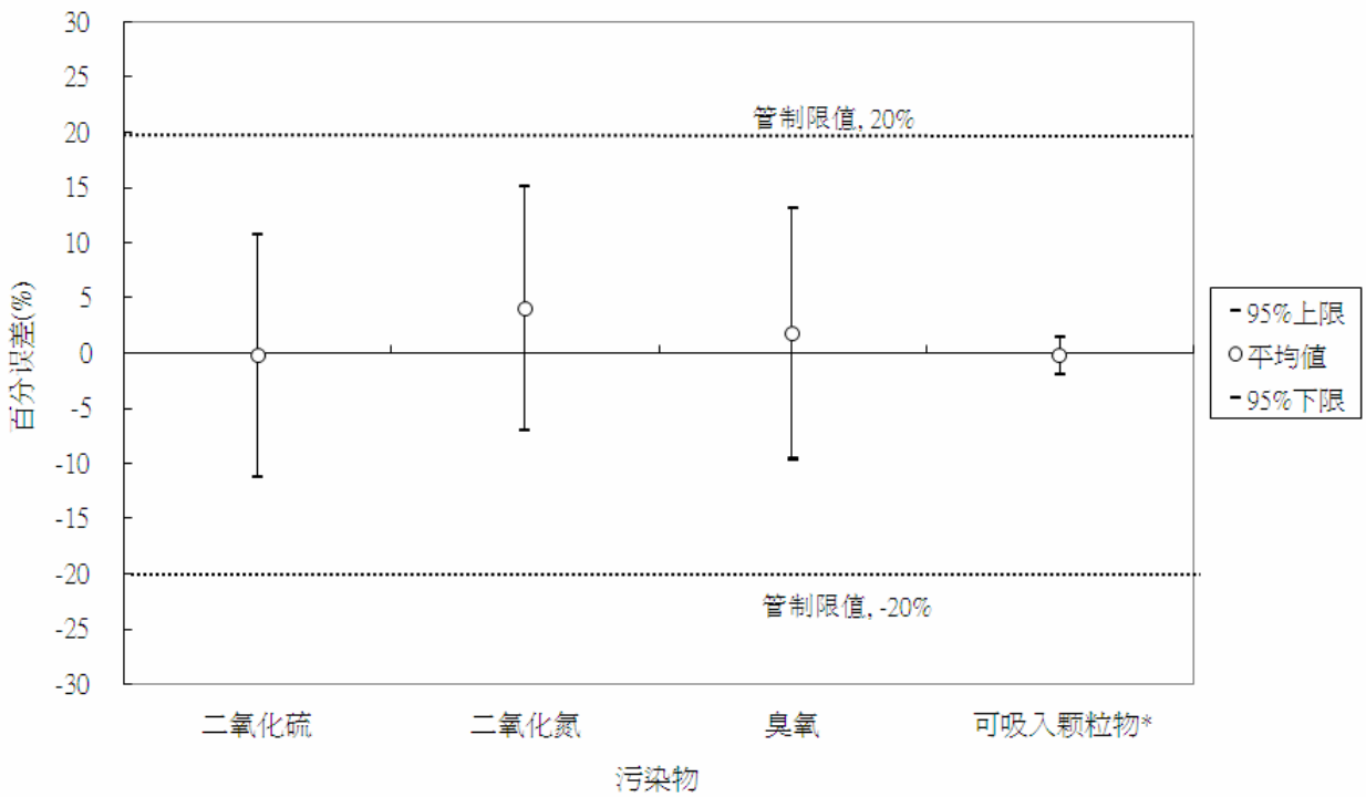
图 3：2008 年粤港珠江三角洲区域空气监控网络的精确度
