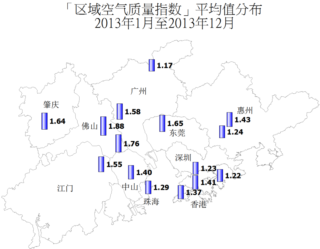
图 11：监控网络内各监测子站的区域空气质量指数平均值分布
