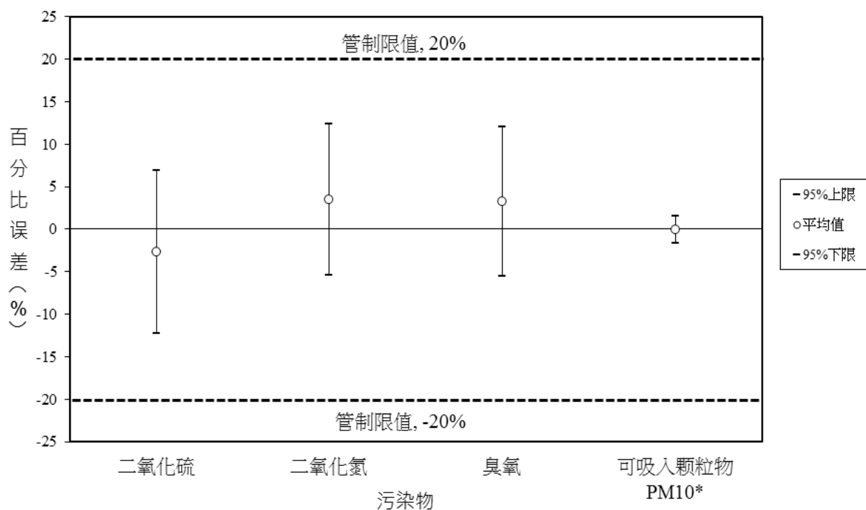
图 3：2013 年粤港澳大湾区区域空气监控网络的精确度
