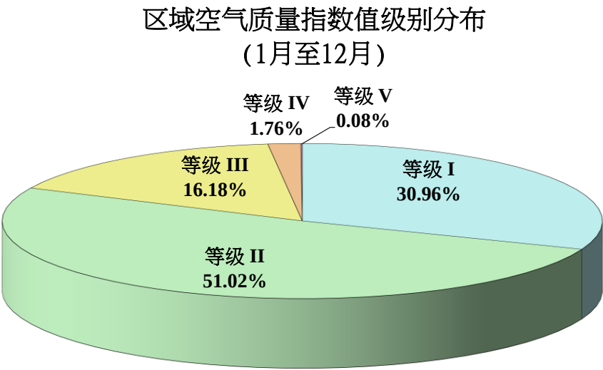
图 10：区域空气监控网络的区域空气质量指数值级别分布
