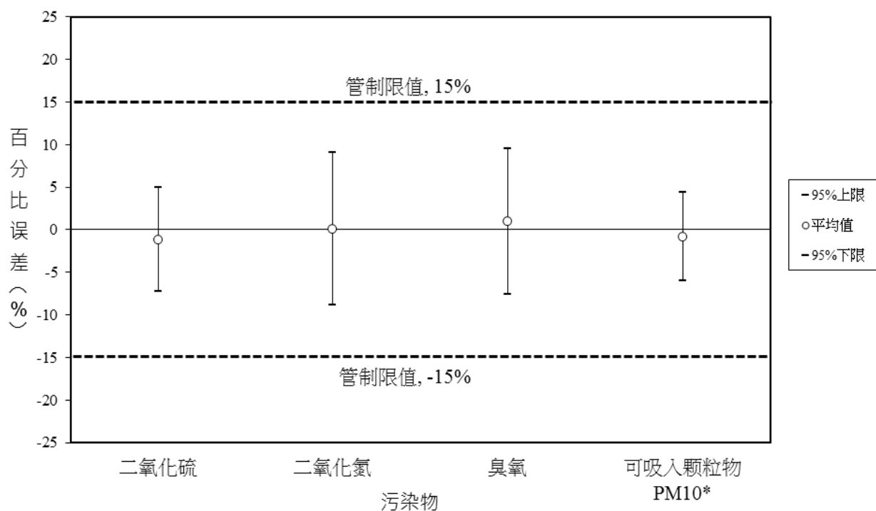
图 2：2013 年粤港澳大湾区区域空气监控网络的准确度
