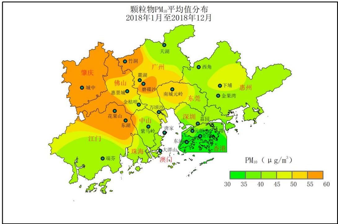
图 9：监测网络颗粒物 PM_{10} 浓度年平均值空间分布
