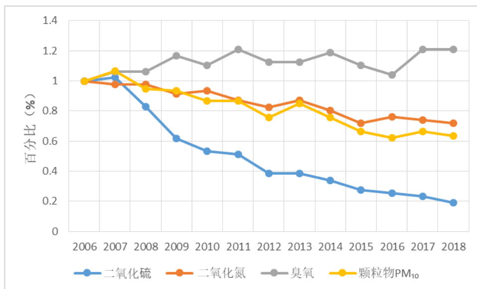
图 12：监测网络污染物浓度年平均值趋势变化
