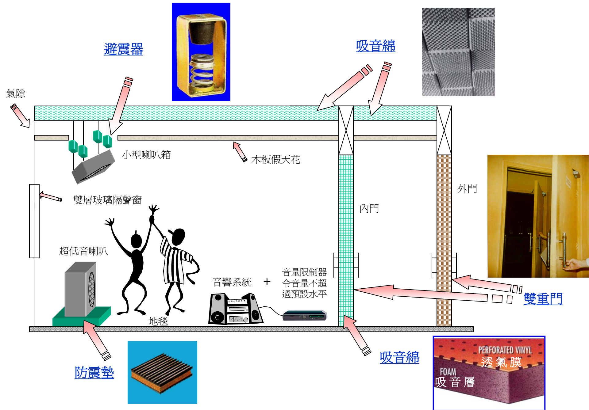
卡拉OK、的士高和酒吧可採用的噪音消減措施
